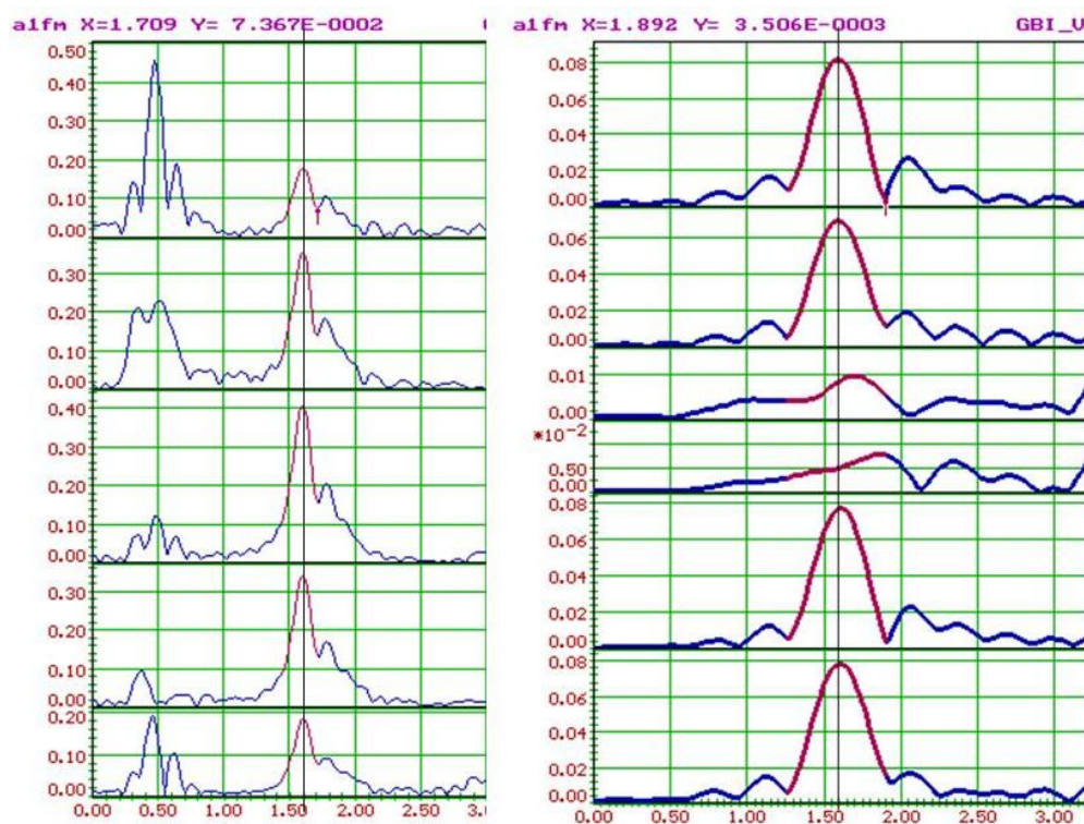
Рисунок 7. Модули спектров колебаний оболочки на частоте 1,59 Гц (2004 г.) и 1,60 Гц (2010 г.)
